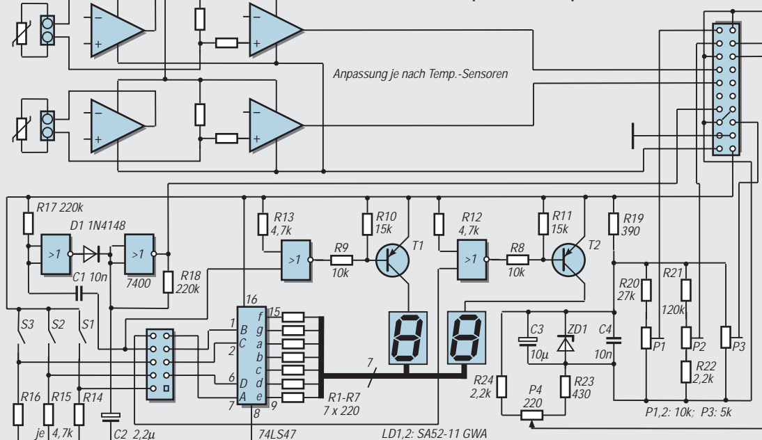
Bild 4: Stromlaufplan der Deckplatine
