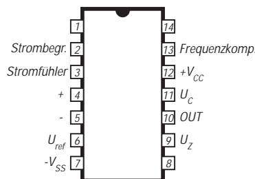
Bild 13: Anschlußschema 7
