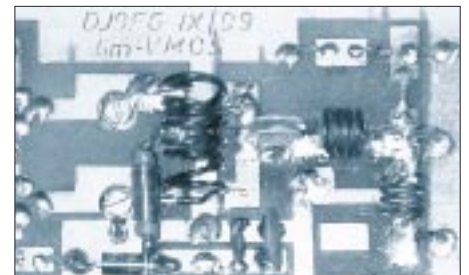
Bild 10: Blick auf den Ausgangsschwingkreis L1/L2 und die Draindrossel Dr
