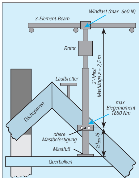
Bild 2: Prinzipische Skizze der Mastbefestigung für eine drehbare Antenne ohne Abspannung am Dachstuhl. Freie Zugänglichkeit des Laufsteges zum Schornstein ist eine Selbstverständlichkeit. Nach [4] darf ein Mastrohr oberhalb des Rotors maximal 1 m lang sein, wenn kein Oberlager zum Einsatz kommt.
