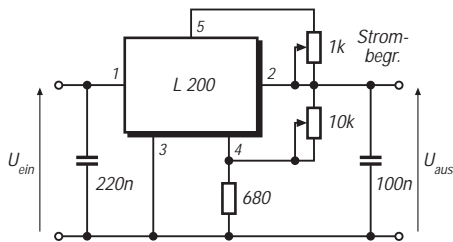
Bild 17: Standardschaltung mit Strombegrenzung (L200)
